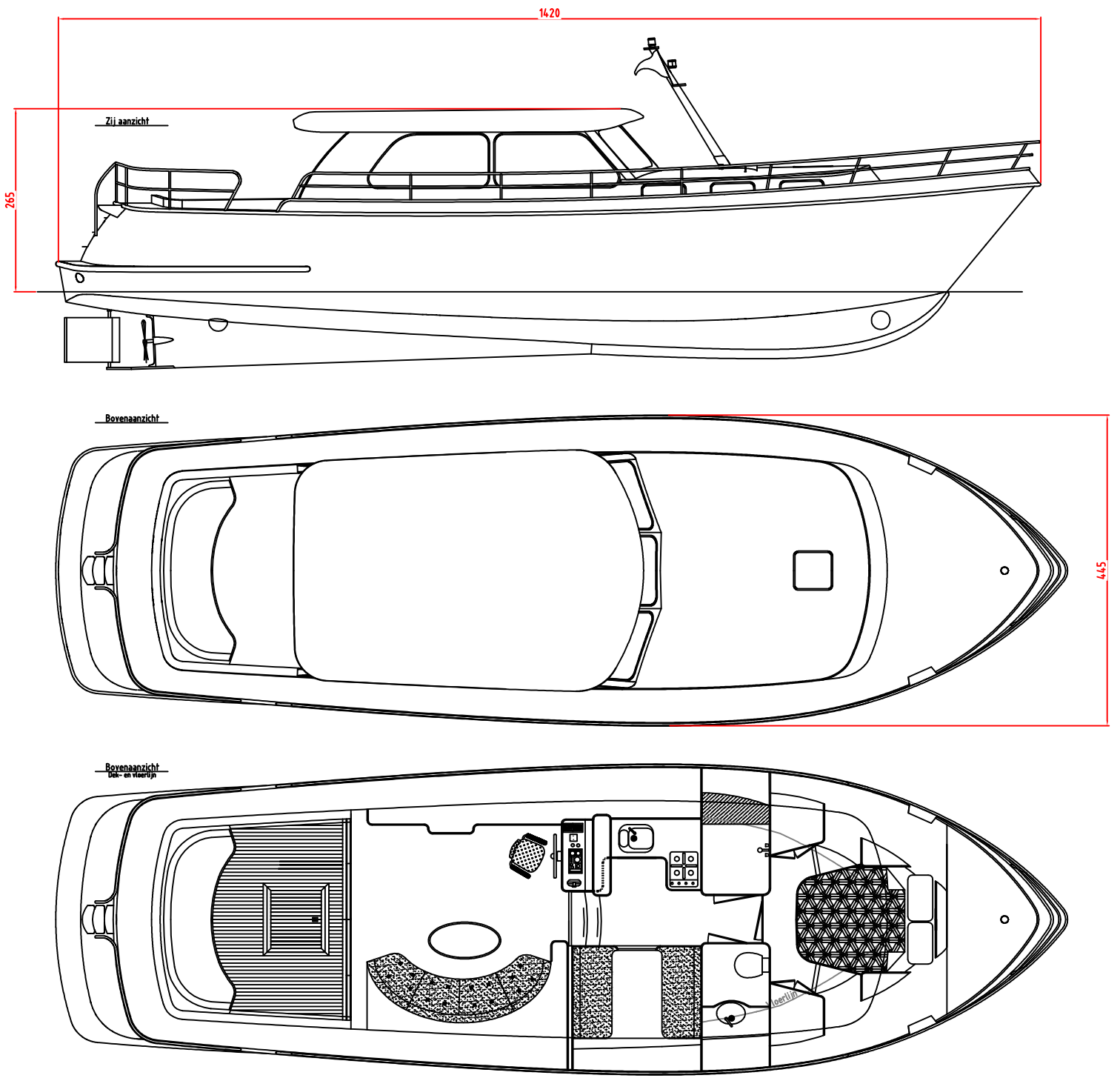
Indelingsmogelijkheid Pikmeerkruiser 48 DC
